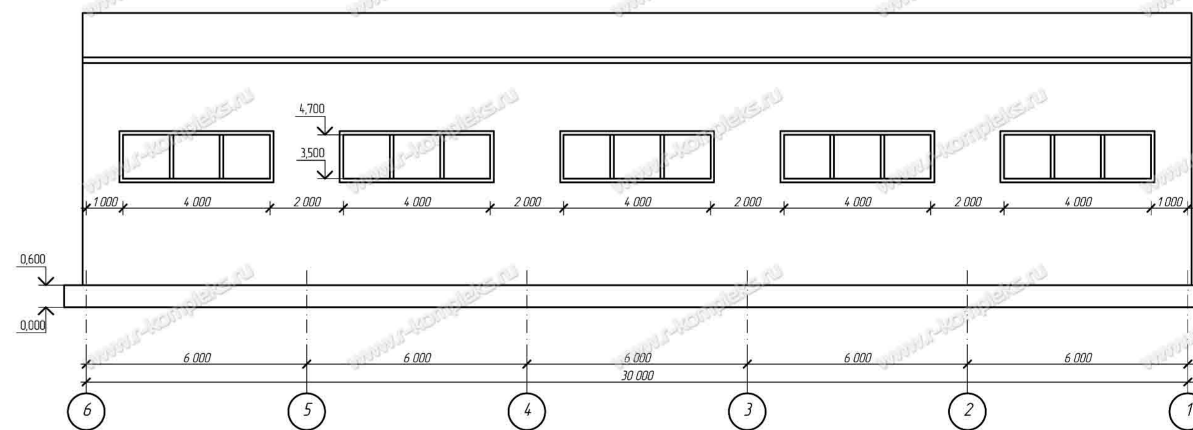
Фасад по оси Д
